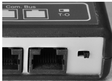
Xcom-232i-Terminierung deaktiviert (O-Stellung)
