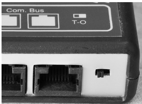
Xcom-232i-Terminierung aktiviert (T-Stellung)
