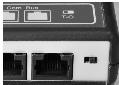
BSP-Terminierung deaktiviert (O-Stellung)
